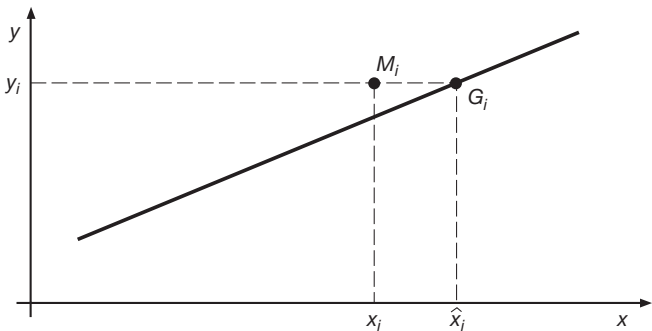
Figure 3.5 – Interprétation géométrique de la droite des moindres carrés \mathbb{D}'
