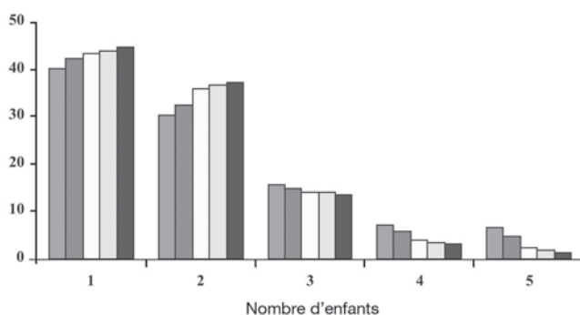
Diagrammes en bâtons juxtaposés
