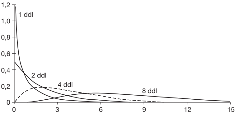
Figure 7.12 – Densités de quelques lois de khi-deux (à 1, 2, 4 et 8 ddl)
