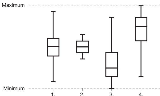
Figure 1.19 – Quelques types de boîtes de distribution : 1. Distribution symétrique 2. Distribution peu dispersée 3. Distribution étalée vers les valeurs élevées 4. Distribution étalée vers les valeurs faibles
