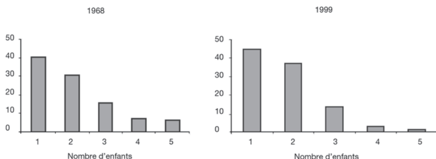
Diagrammes en bâtons juxtaposés
