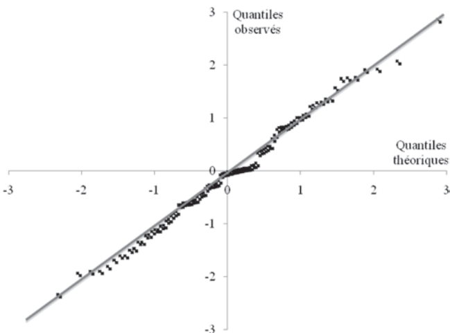
Figure 1 – Diagramme Quantile-Quantile obtenu pour les 100 valeurs
