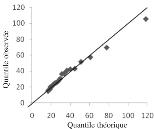
Figure 7.24 – Diagramme Quantile-Quantile (unité : milliards d'euros) Loi de Pareto de paramètres \alpha = 1,646 et x_0 = 16\,774
