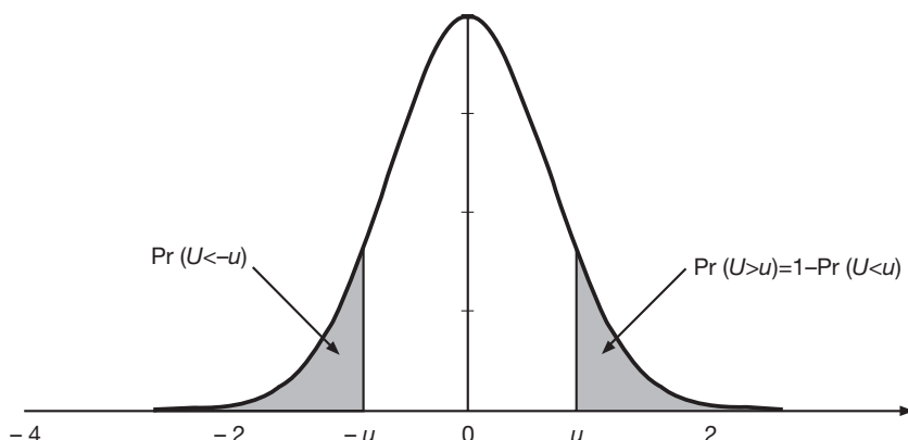
Figure 7.7 – Calcul de probabilité d'intervalles symétriques pour une loi de Gauss centrée réduite
