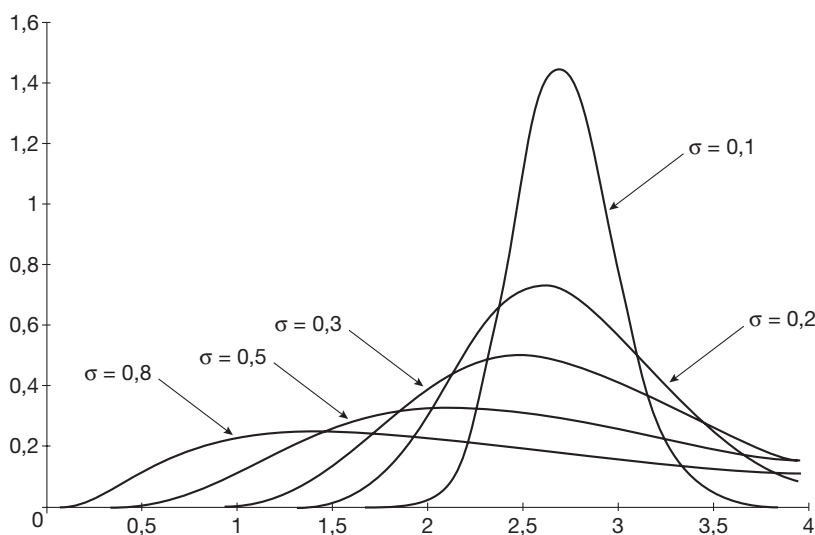
Figure 7.19 – Asymétrie de la loi log-normale \mathcal{LN}(0, 1, \sigma) en fonction de \sigma
