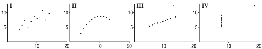
Figure 3.7 – Extrait de F. J. Anscombe : Graphs in Statistical Analysis, adapté avec la permission de The American Statistician, 27 (February 1973), 17-21, American Statistician Association
